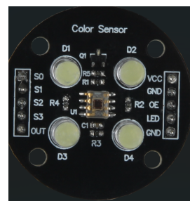
Fig. 21. Color Sensor
